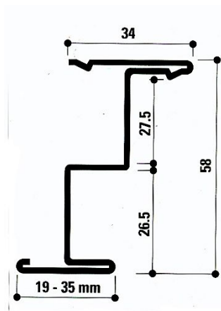
Perfil Z 151-152 de Chicago Metallic®
