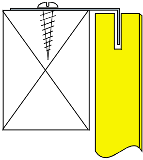
Det S1: EL-30 perfil.
