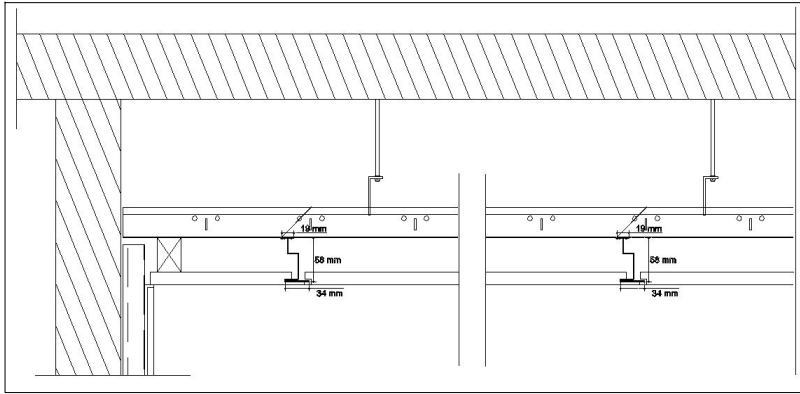
Detalle falso techo registrable con perfilera Chicago Metallic®
