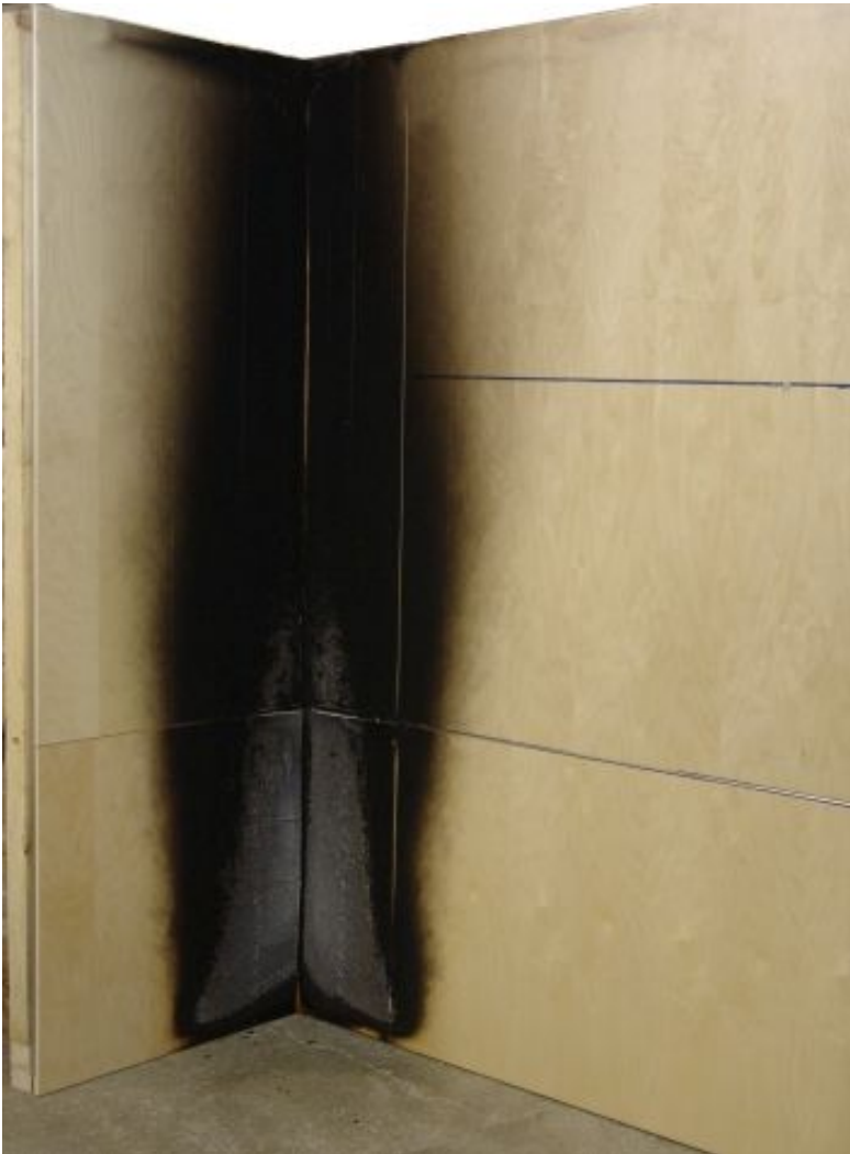
Panel Elam en SBI (Prueba contra el fuego)
