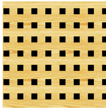
Hål 12x12 mm, cc 32,5 mm, hålärea 14 %.
