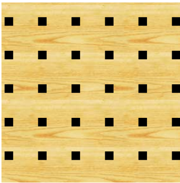
Hål 10x10 mm, cc 45 mm, hålärea 5 %.
